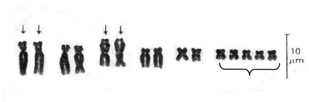
Figura 2.3 - Cromosomas B en Puschkinia libanotica .
